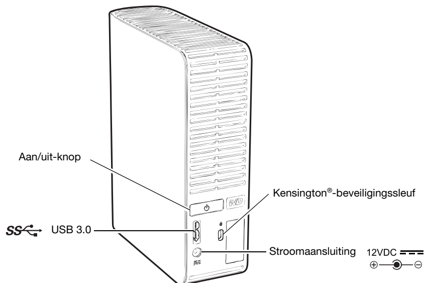
Afbeelding 3. Achterzijde van de My Book Essential-schijf
