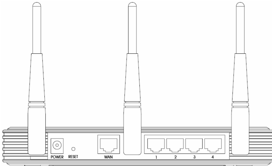
Bild 1-2 Geräterückseite
